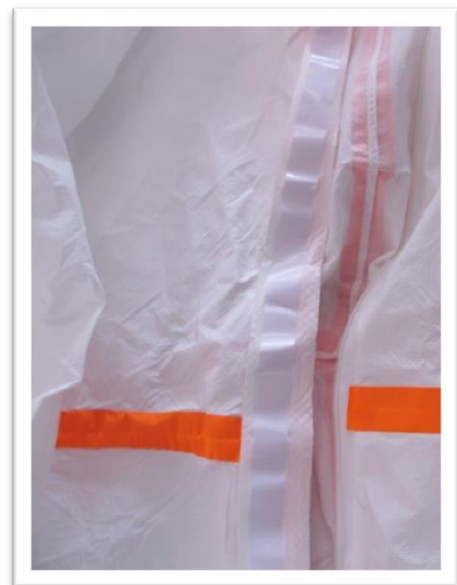
Detalle de solapa adhesiva para cubrir la cremallera y de esta manera mejorar la impermeabilización del traje.
